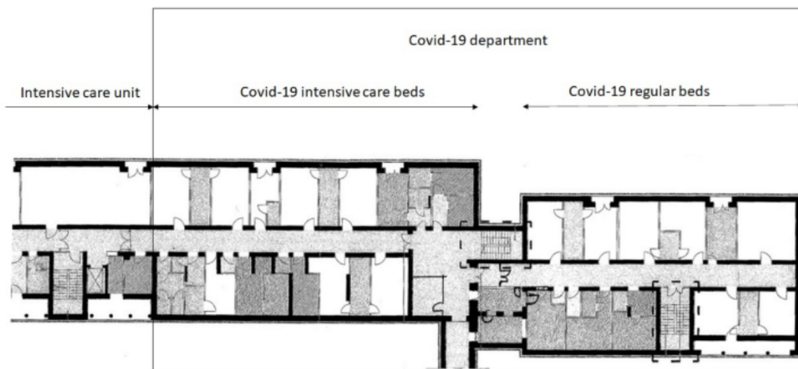
Figur 4.5 Planskisse av ortopedisk sengeområde som ble ombygd til sengeområde for covid-19-pasienter. Kilde: Białoszewski, A. Z. et al. 2021
