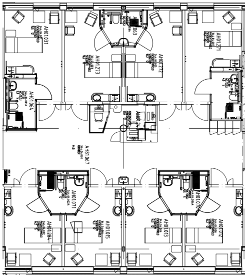
Figur 4.28 Illustrasjon over sengetun med 8 ensengsrom, arbeidsstasjon og lagerskap, St. Olavs hospital, Øya: Kilde: Team St. Olav arkitekter
