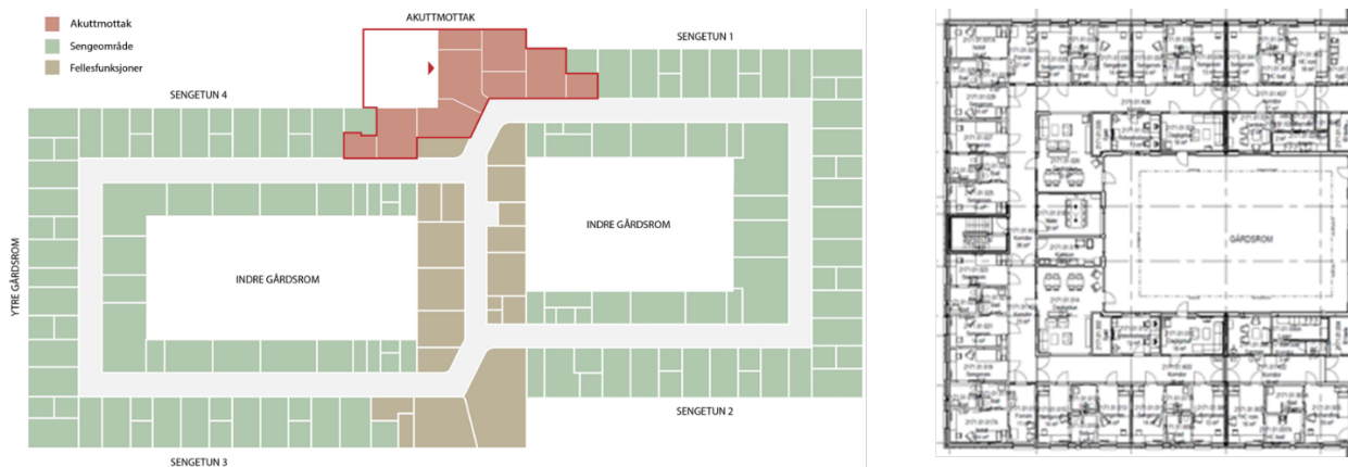
Figur 4.27 Illustrasjon over døgnområdene og akuttmottaket, samt utsnitt av to tun ved Akuttbygget Østmarka, St. Olavs hospital. Kilde: Nordic Office of Architecture og SLA 28.11.2014. Bearbeidet av sykehusbygg HF 2023
